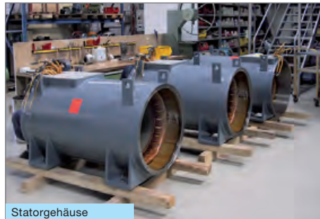
Statorgehäuse
